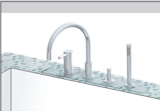
B - BORDO V-BOX CON PIASTRA RIVESTITA. OPTIONAL: SISTEMA DI PRE-INSTALLAZIONE (012/6) B - BORDO V-BOX WITH FACED PLATE. OPTIONAL: PRE-INSTALLATION SYSTEM (012/6) C - BORDO V-BOX CON PIASTRA RIVESTITA. OPTIONAL: SISTEMA DI PRE-INSTALLAZIONE (012/6) E VASCHETTA DI RACCOLTA (012/7) C - BORDO V-BOX WITH FACED PLATE. OPTIONAL: PRE-INSTALLATION SYSTEM (012/6) AND COLLECTION CASE (012/7)
