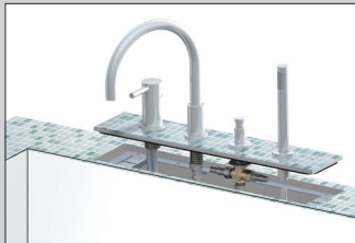
B - BORDO V-BOX CON PIASTRA RIVESTITA. OPTIONAL: SISTEMA DI PRE-INSTALLAZIONE (012/6) B - BORDO V-BOX WITH FACED PLATE. OPTIONAL: PRE-INSTALLATION SYSTEM (012/6) C - BORDO V-BOX CON PIASTRA RIVESTITA. OPTIONAL: SISTEMA DI PRE-INSTALLAZIONE (012/6) E VASCHETTA DI RACCOLTA (012/7) C - BORDO V-BOX WITH FACED PLATE. OPTIONAL: PRE-INSTALLATION SYSTEM (012/6) AND COLLECTION CASE (012/7)
