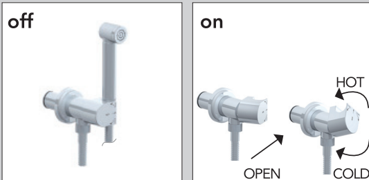
GANCIO DOCCETTA BIDET COMPLETO CON MISCELATORE INTEGRATO COMPLETE HOOK HAND SHOWER BIDET WITH INTEGRATE MIXER ART. 0403/MI, 0903/MI, 7503/MI, 3303/MI, 0303/MI, 1403/MI
