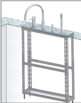
B - BORDO V-BOX CON PIASTRA RIVESTITA. OPTIONAL: SISTEMA DI PRE-INSTALLAZIONE (012/6) B - BORDO V-BOX WITH FACED PLATE. OPTIONAL: PRE-INSTALLATION SYSTEM (012/6) C - BORDO V-BOX CON PIASTRA RIVESTITA. OPTIONAL: SISTEMA DI PRE-INSTALLAZIONE (012/6) E VASCHETTA DI RACCOLTA (012/7) C - BORDO V-BOX WITH FACED PLATE. OPTIONAL: PRE-INSTALLATION SYSTEM (012/6) AND COLLECTION CASE (012/7)
