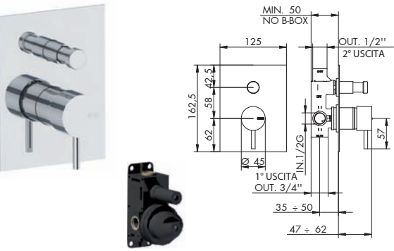
INCASSO UNIVERSALE CON B-BOX
