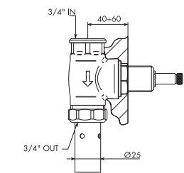
Art. 8840/E Parti esterne per passo rapido External parts for built-in rapid flow cock 01-8840/E cromato
